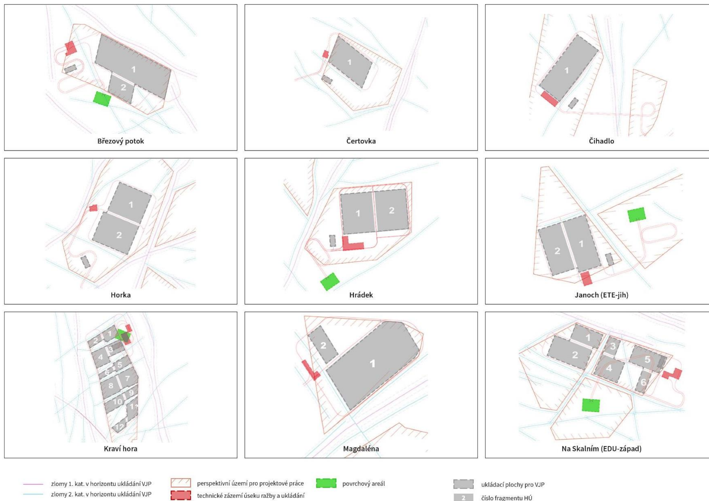
Obr.: 16 Schéma fragmentace podzemní části HÚ území dle (Butovič et al. 2020)
