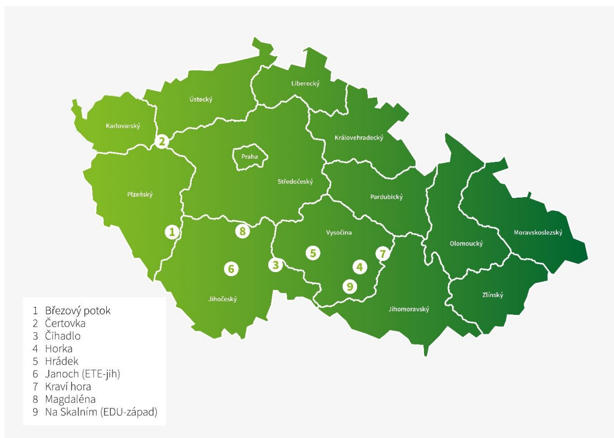
Obr.: 2 Potenciální lokality hlubinného úložiště v letech 2014-2020
